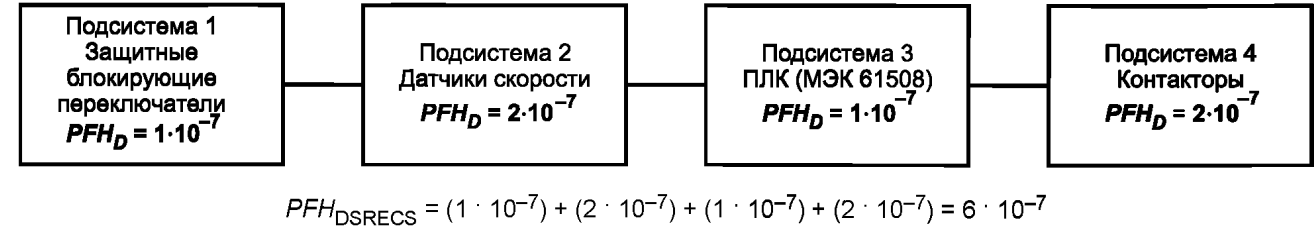
Рисунок В.8 — Оценка PFH_D для СБЭСУ
